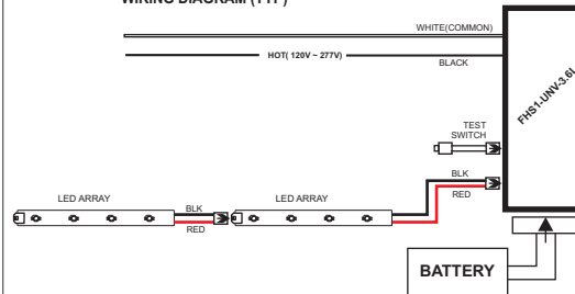
WIRING DIAGRAM (TYP)
